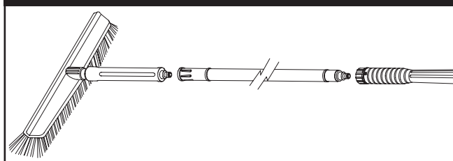
Figura 30 - Conexión del Cepillo de Suelo a la Pistola Rociadora
